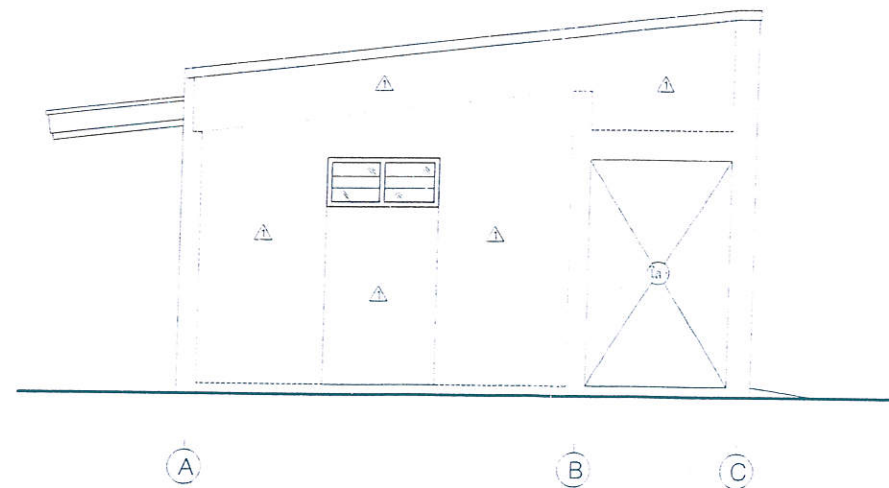
รูปด้าน ② SCALE 1:75
